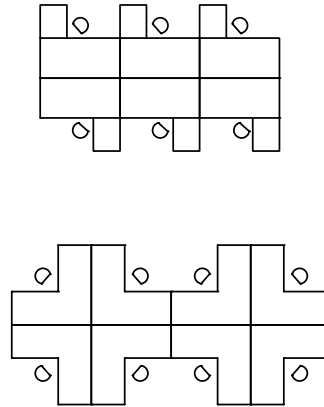
Length 1200-2400 Width 600-900
