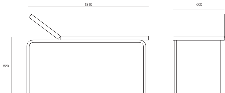
Tubular Frame
